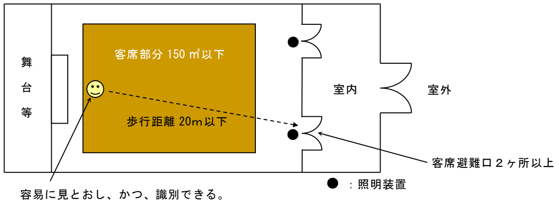
第17-17図 劇場等の誘導灯の設置緩和例
