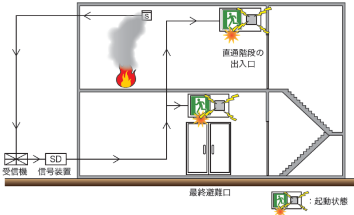
第17-30図 点滅形誘導灯等の起動
