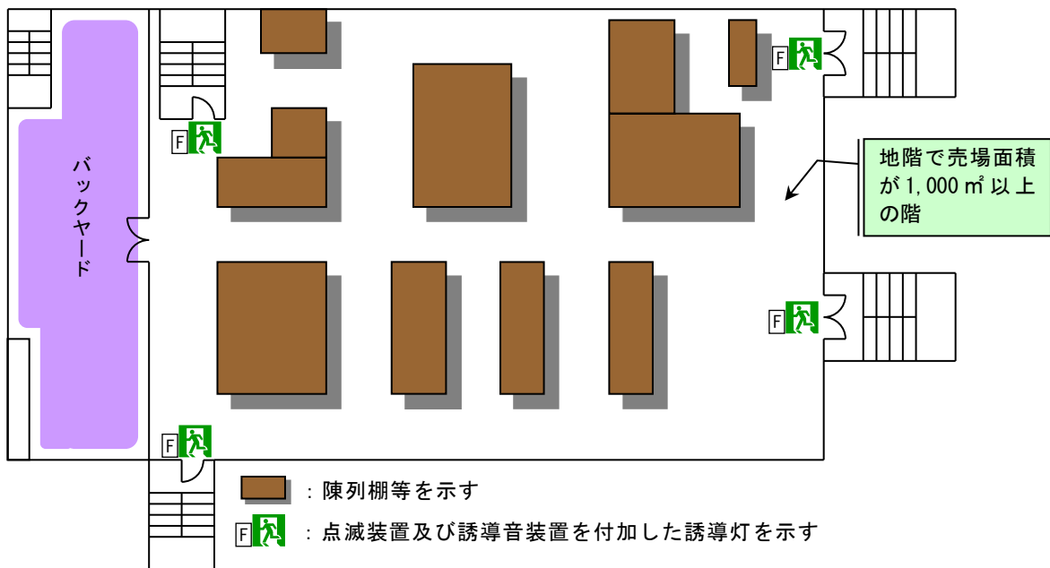
第17-29図 点滅形誘導灯等の設置例
