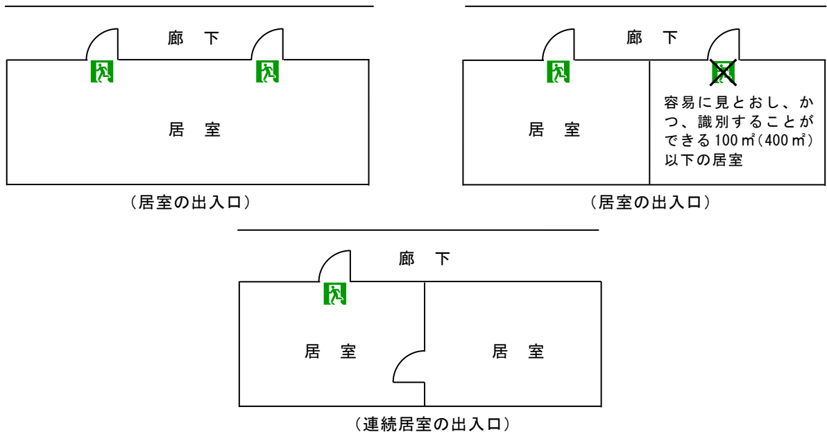
第17-8図 居室から廊下へ通ずる出入口の例
