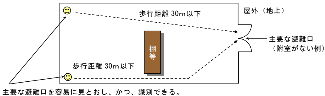
第17-56図 誘導標識の設置を要しない例
