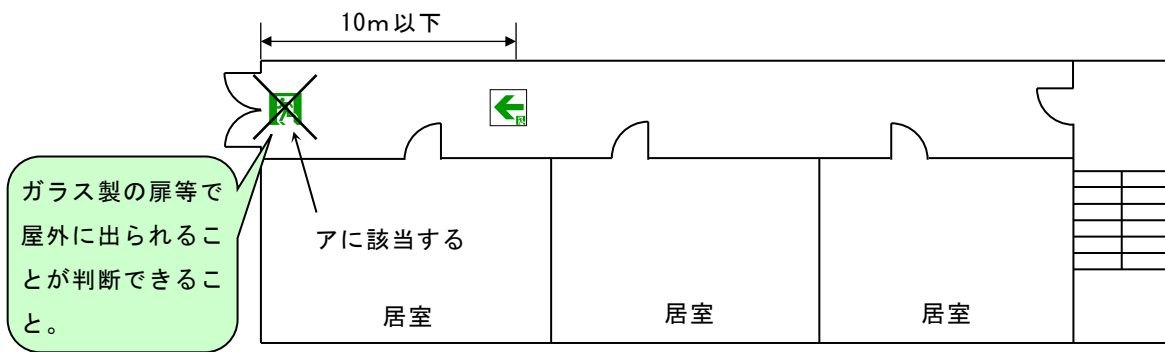
第17-21図 避難口誘導灯の設置緩和例
