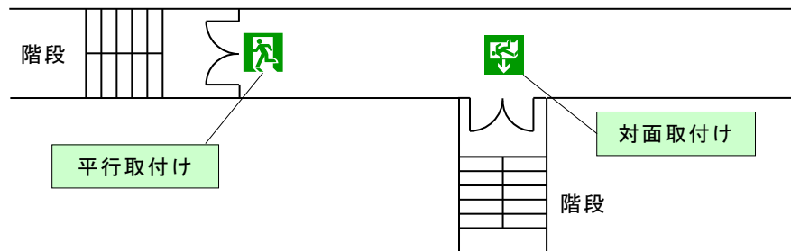
第17-12図 避難口誘導灯の設置例
