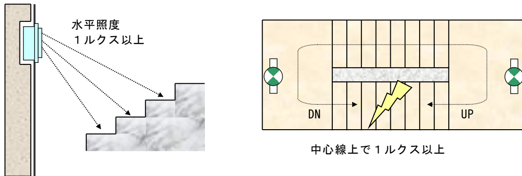
第17-51図 階段通路誘導灯の設置例
