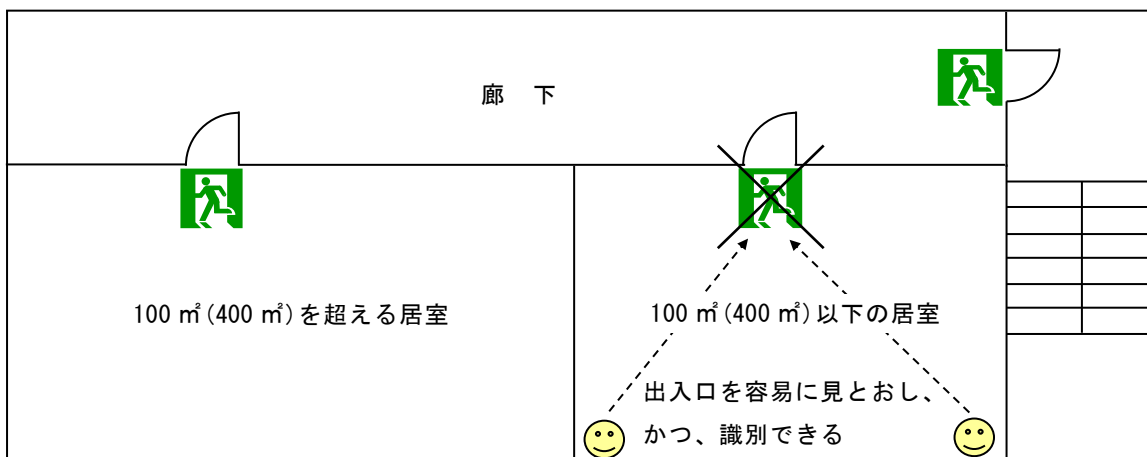
第17-16図 居室から廊下へ通ずる出入口の例
