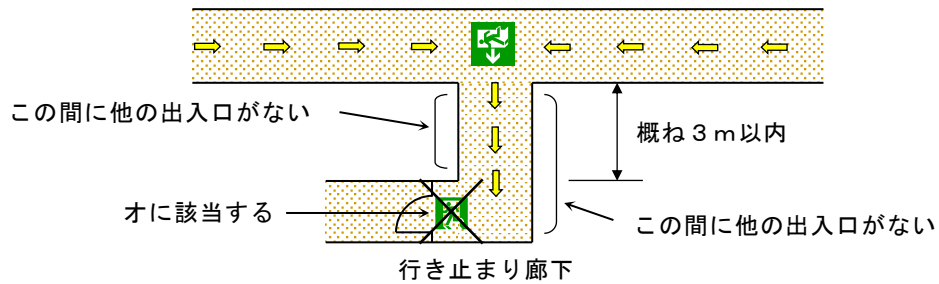
第17-24図 避難口誘導灯の設置緩和例
