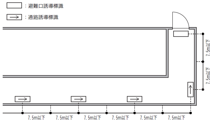
第17-55図 誘導標識の設置例
