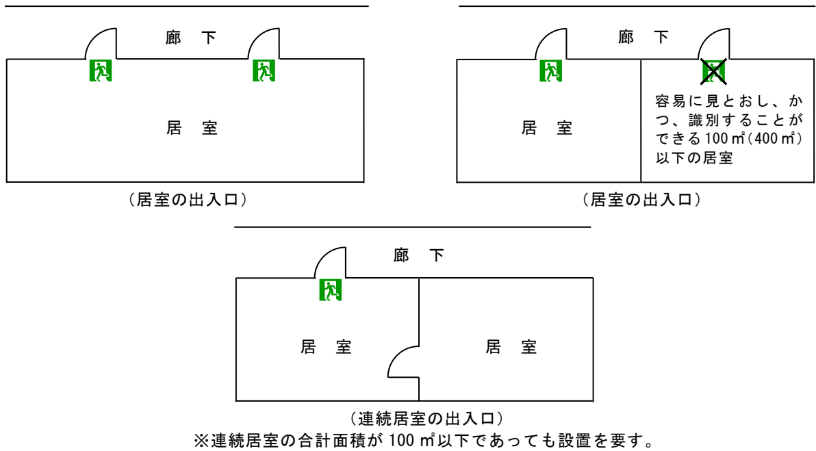
第17-8図 居室から廊下へ通ずる出入口の例
