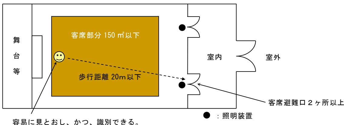
第17-17図 劇場等の誘導灯の設置緩和例
