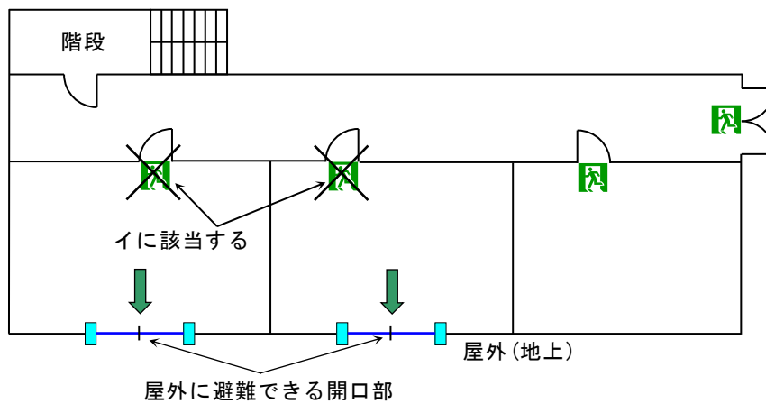
第17-22図 避難口誘導灯の設置緩和例
