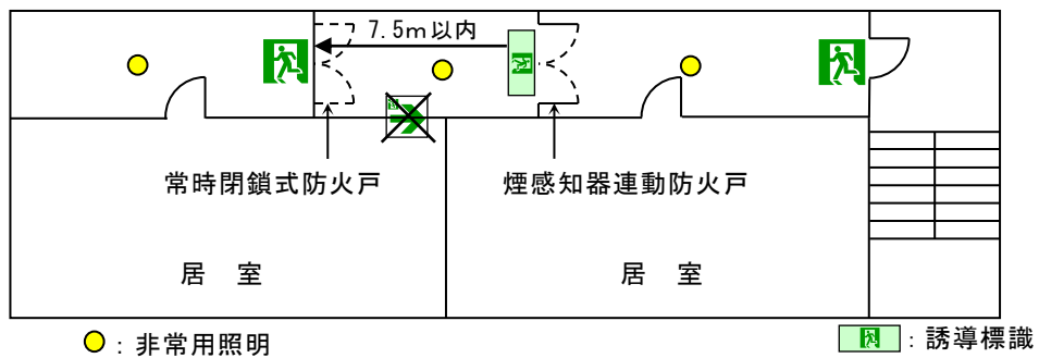
第17-9図 廊下の途中にある防火戸の例
