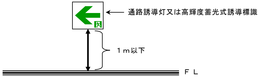
第17-41図 (2)項ニにおける通路誘導灯又は高輝度蓄光式誘導標の設置高さの例
