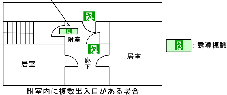
第17-7図 直通階段の出入口の例
