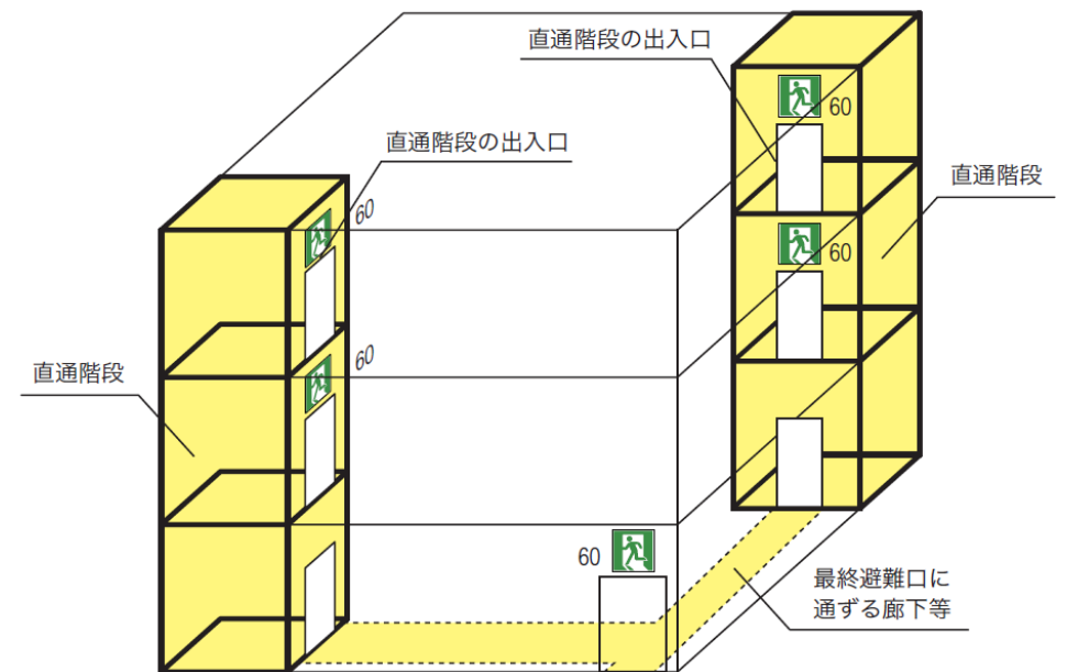
第17-57図 主要な避難経路に設ける誘導灯
