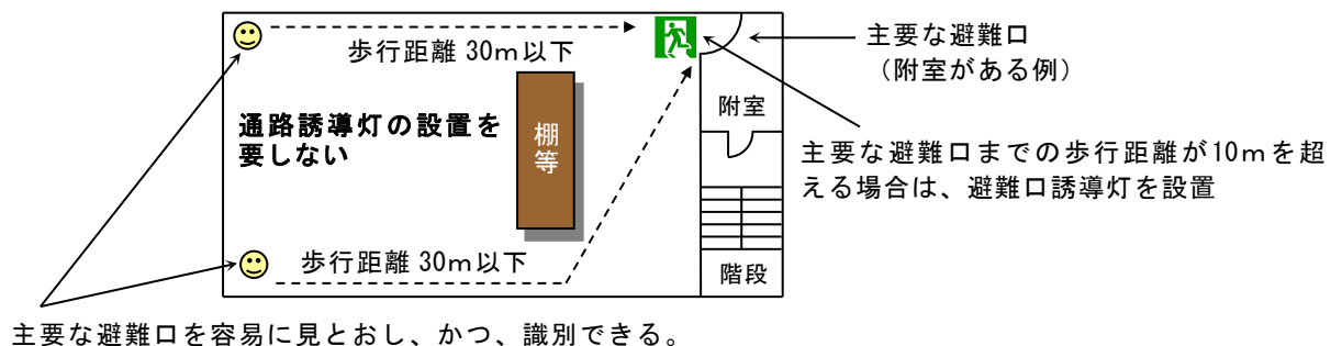
第17-49図 通路誘導灯の設置を要しない例（避難階以外の階）
