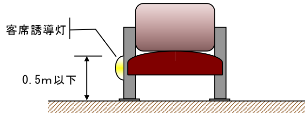
第17-52図 客席誘導灯の設置例
