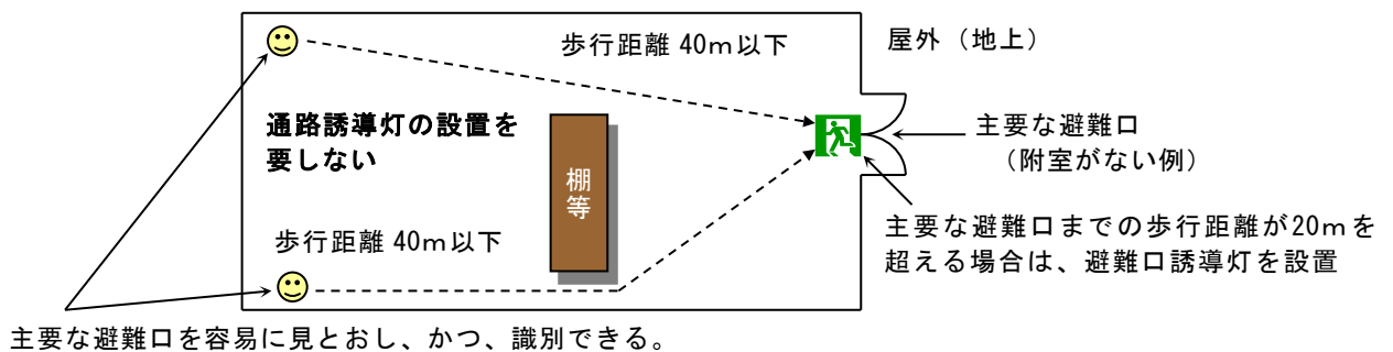
第17-48図 通路誘導灯の設置を要しない例（避難階）
