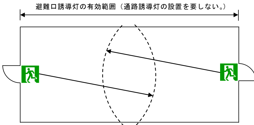
第17-37図 避難口誘導灯の設置により誘導灯の有効範囲として緩和される場合の例
