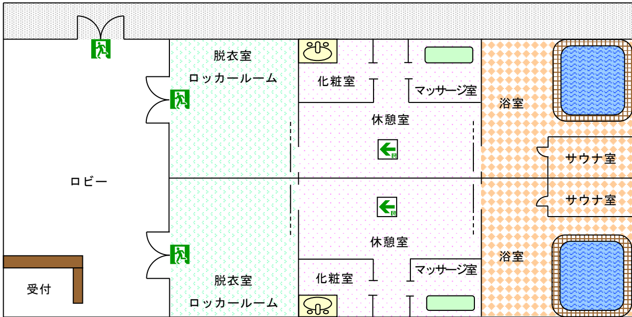
第17-40図 誘導灯の設置例
