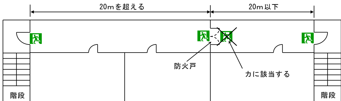
第17-25図 避難口誘導灯の設置緩和例
