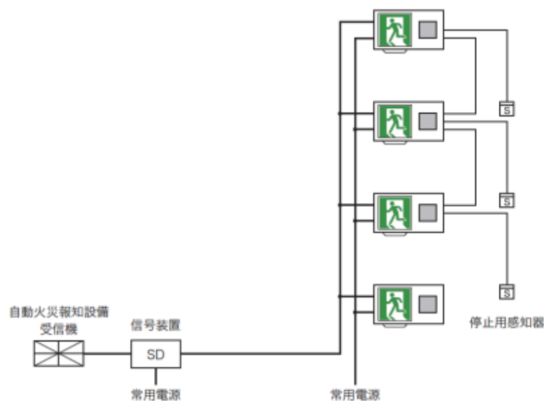
第17-28図 点滅機能及び音声誘導機能を付加した誘導灯の主な構成図
