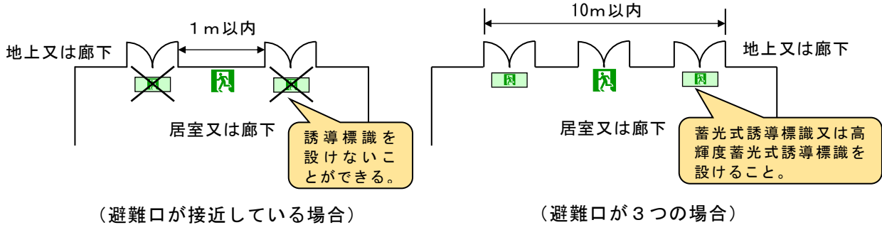
第17-26図 避難口誘導灯の緩和例
