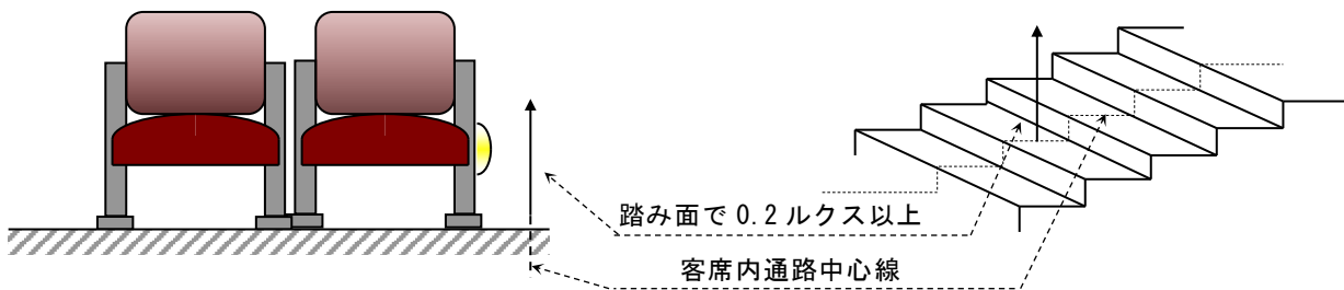
第17-53図 水平照度
