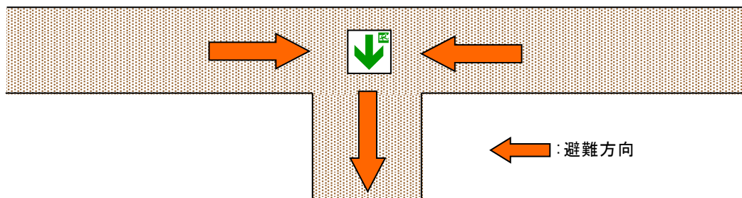
第17-38図 床又は天井に通路誘導灯を設置した場合の設置例
