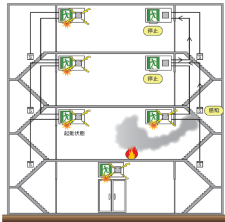
第17-31図 点滅形誘導灯等の消灯
