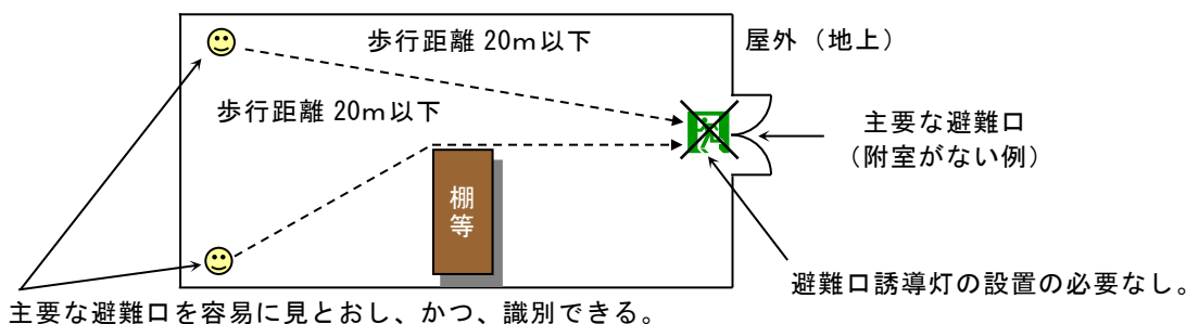
第17-14図 避難口誘導灯の設置を要しない例(避難階)
