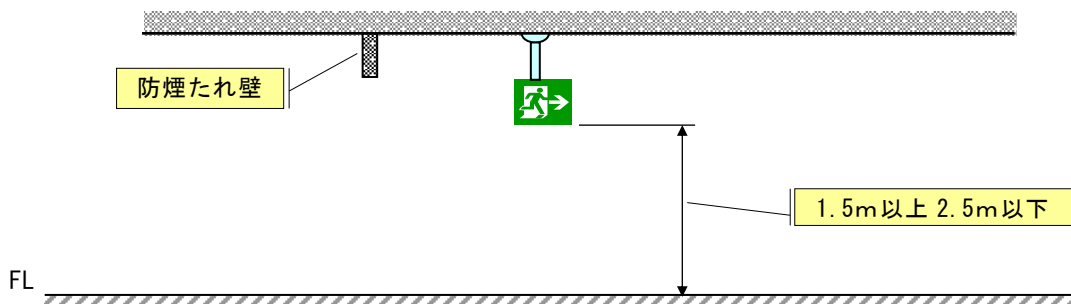
第17-13図 避難口誘導灯の設置高さの例
