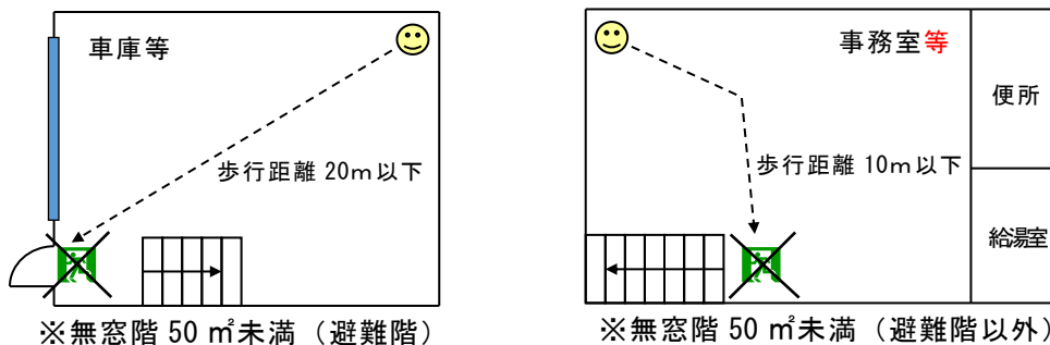
第17-27図 無窓階となる場合の設置緩和例
