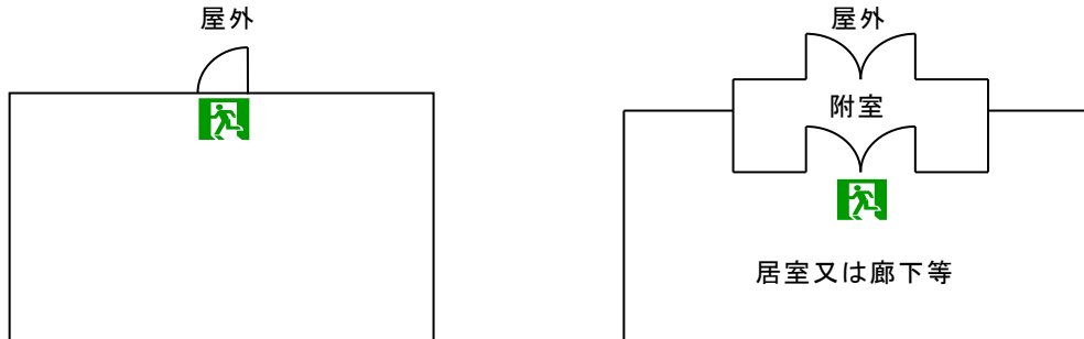
第17-6図 屋内から直接地上へ通ずる出入口の例
