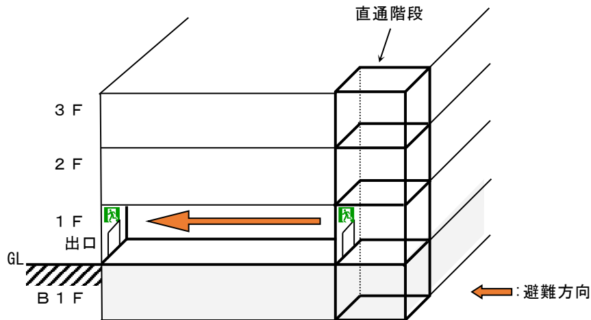
第17-11図 直通階段の階段室から廊下へ通ずる出入口の例
