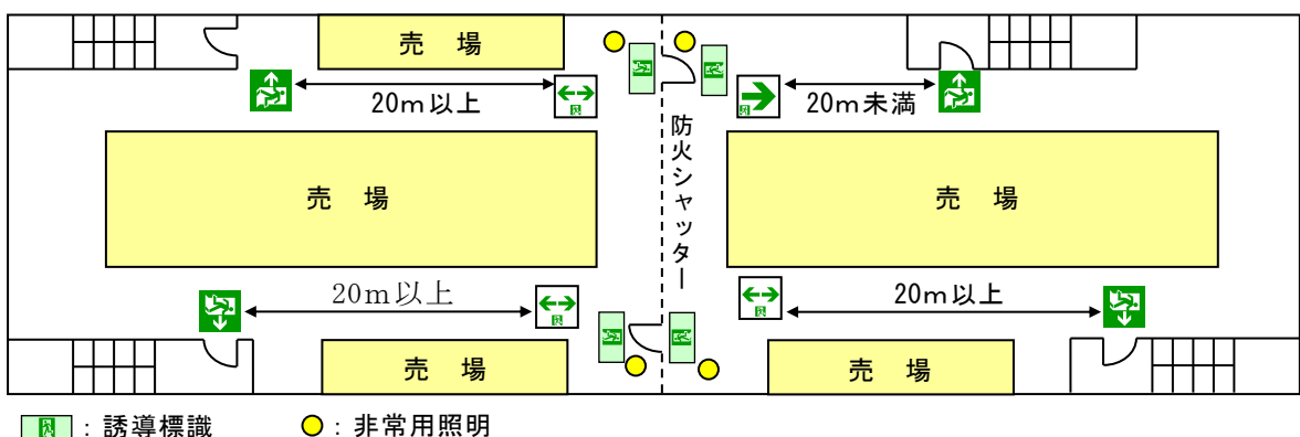
第17-39図 誘導灯の設置例
