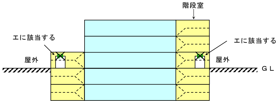
第17-23図 避難口誘導灯の設置緩和例
