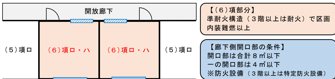
第17-18図 (6)項口及びハの用途に供される居室の区画の例
