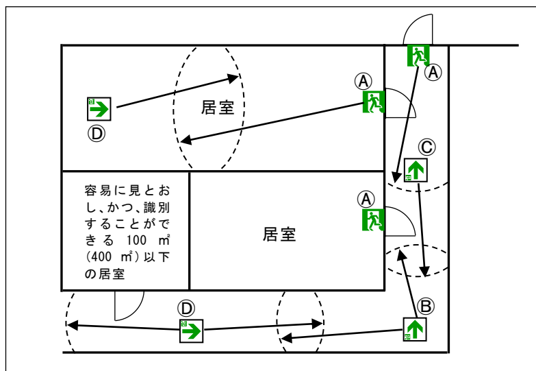
第17-5図 避難口誘導灯及び通路誘導灯を設置する場合の手順
