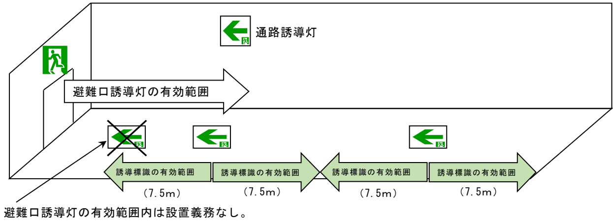
第17-42図 (2)項ニにおける高輝度蓄光式誘導標識の設置例
