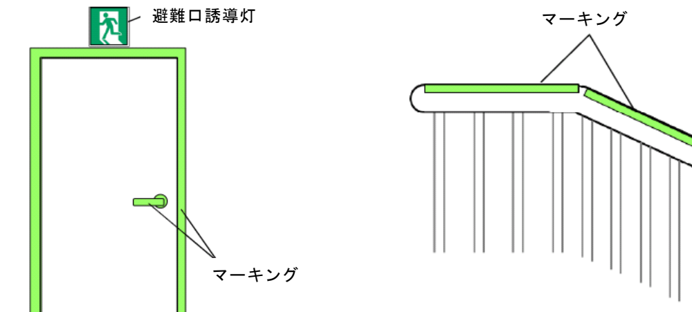
第17-45図 避難口の外周やドアノブ、階段等の手すりをマーキングする標示の設置例
