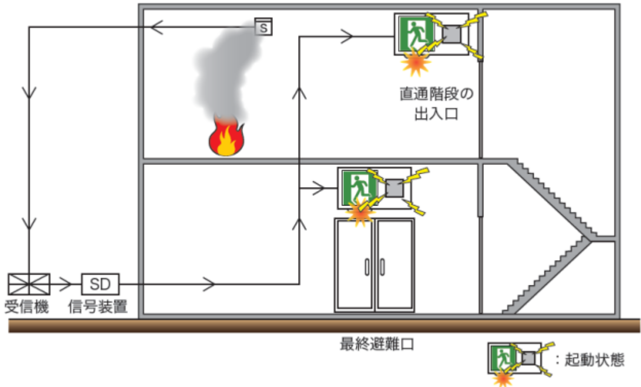
第17-30図 点滅形誘導灯等の起動
