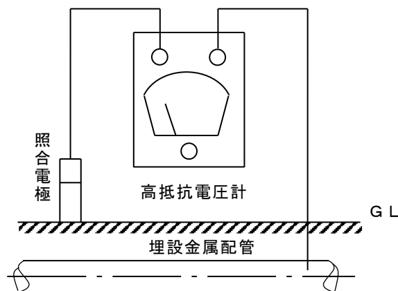
別図第 5 対地電位測定方法
