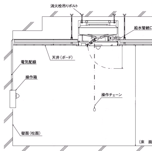
天井設置型消火栓設置例
