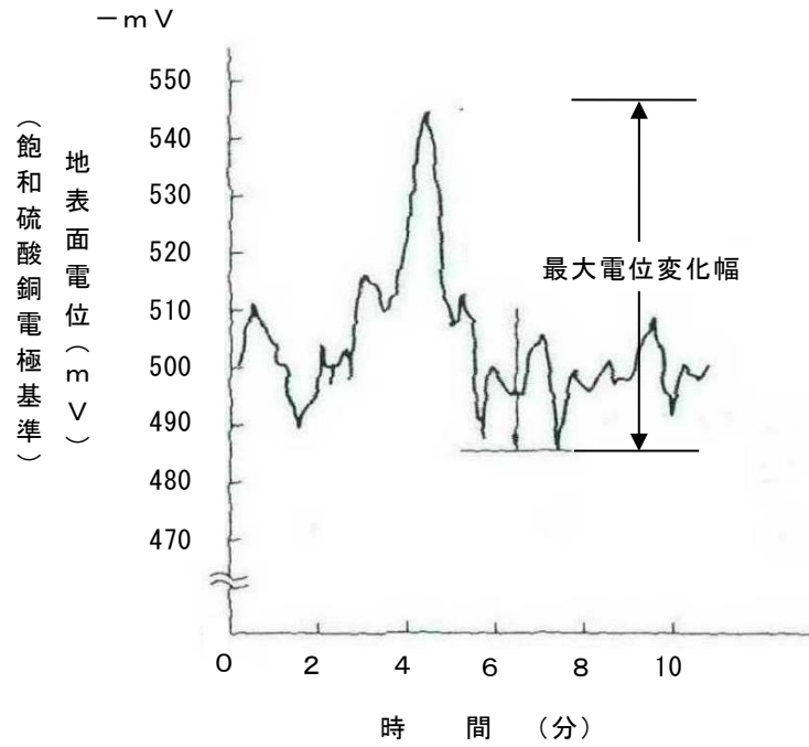
別図第2 対比電位測定例 (電車軌道からの漏れ電流の影響)
