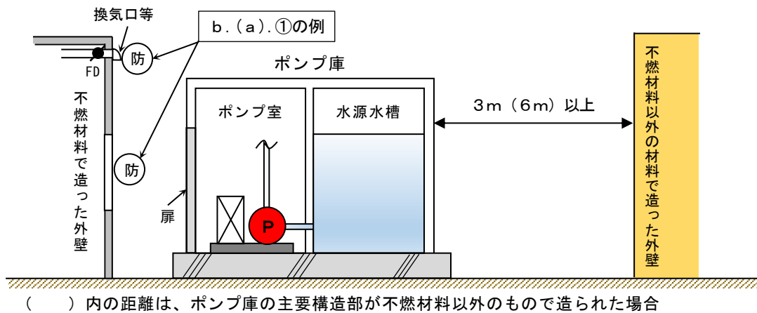
(配置図)
