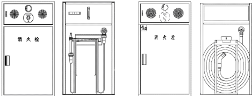
1号消火栓（易操作性1号消火栓を除く。）
