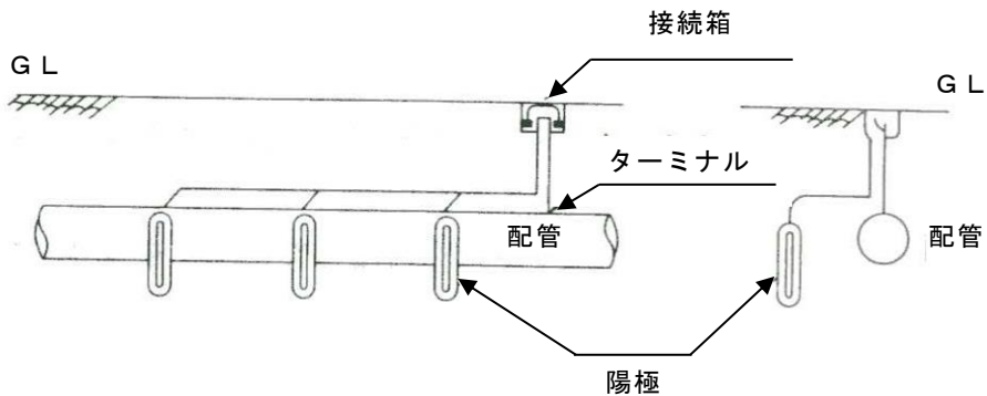
(流電陽極方式の例)
