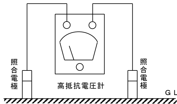
別図第 4 地表面電位こう配測定方法
