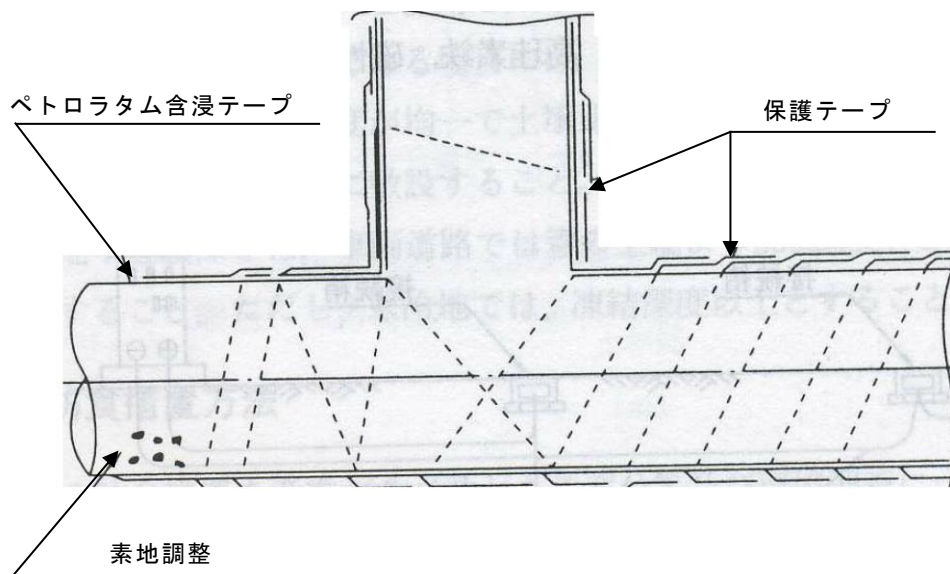
(ペトラタム含浸テープを用いる施工例)
