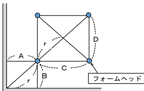
第5-3図 フォームヘッドの平面配置図（ r = 2.1\text{m} の場合）
