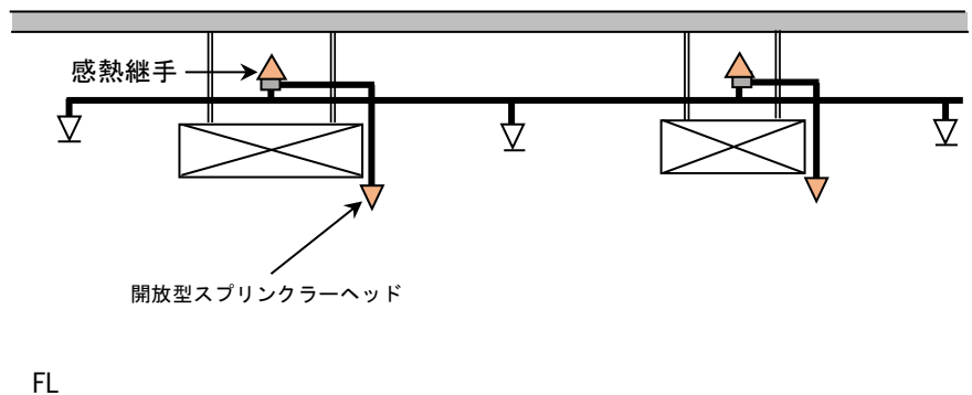
(感熱継手を設ける場合の例)
