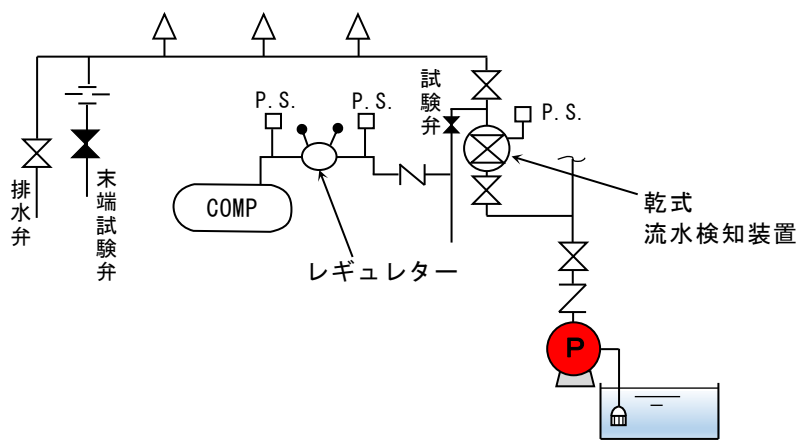
第4-32図 乾式流水検知装置の場合
