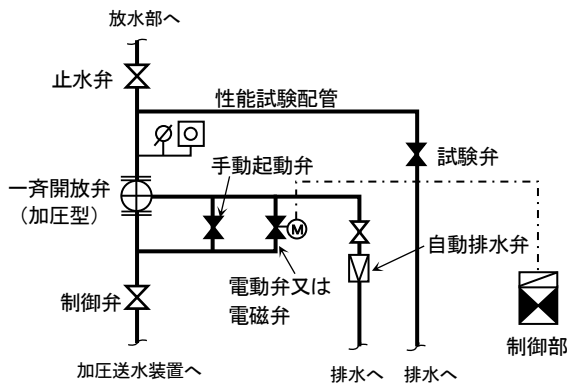
第 4-18図 (加圧方式の一斉開放弁等の廻りの配管図例)
