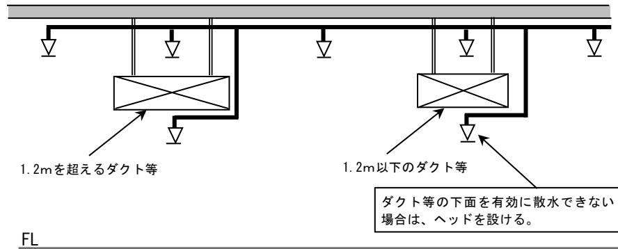
(感熱継手を設けない場合の例)
