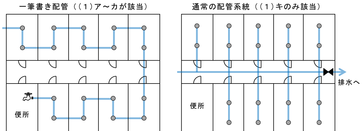
第 4-40図 (一筆書き配管の例)
