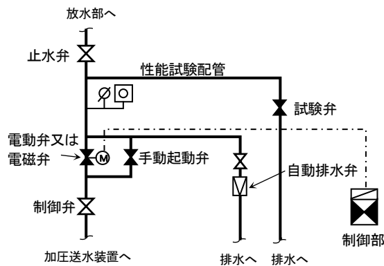
第 4-19図 (電動又は電磁弁方式の廻りの配管図例)
