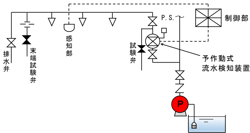
第4-31図 予作動式流水検知装置の場合
