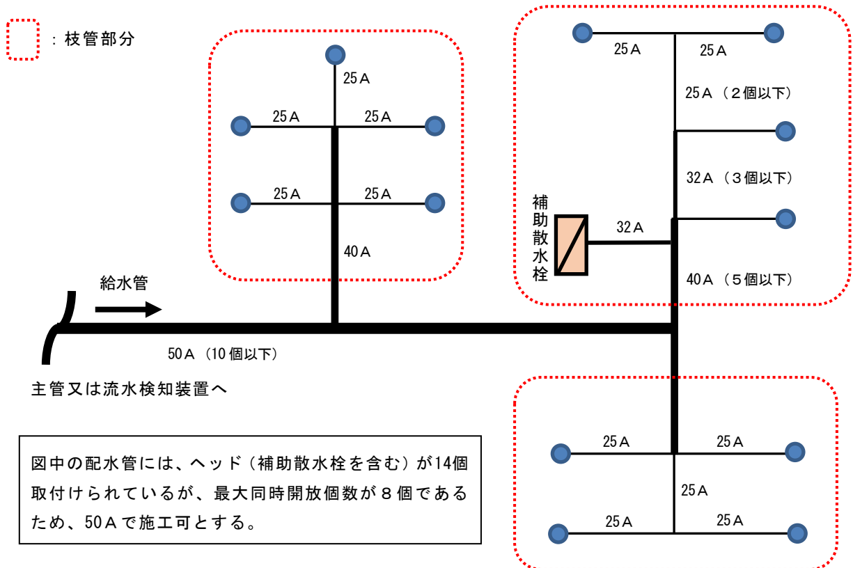
第 4-4 図 配置の設置例：標準型ヘッド(最大同時開放個数 8 個)の場合
