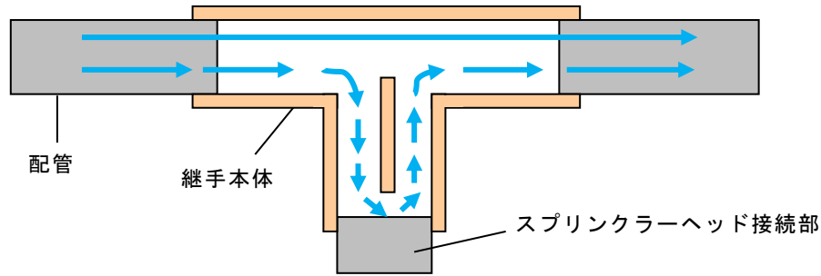
第 4-39図 (停滞防止継手)
