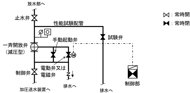
第 4-17図 (減圧方式の一斉開放弁等の廻りの配管図例)
