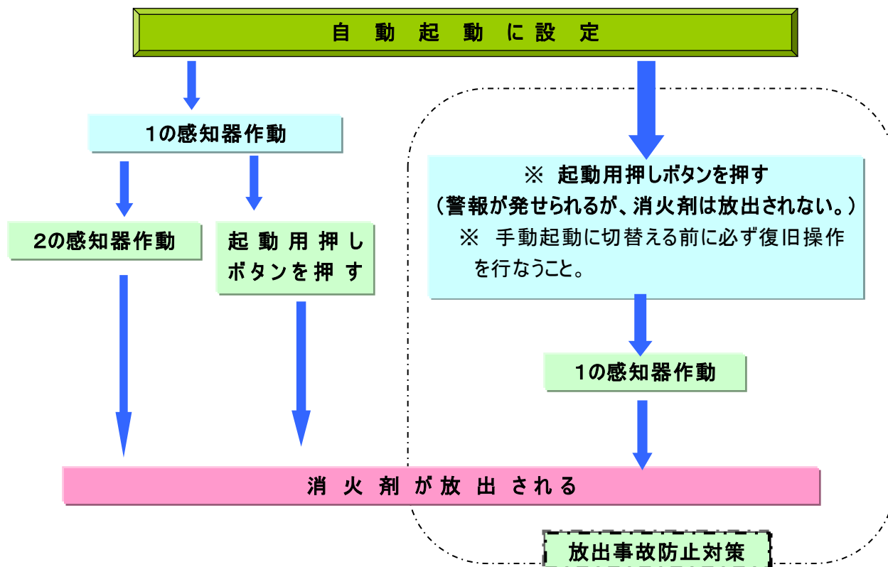
放出事故防止対策システムフロー図
