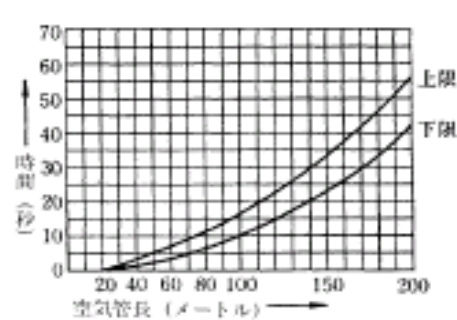
② 空気管の内径が1.5mmの場合
