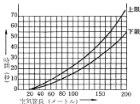
① 空気管の内径が1.4mmの場合
