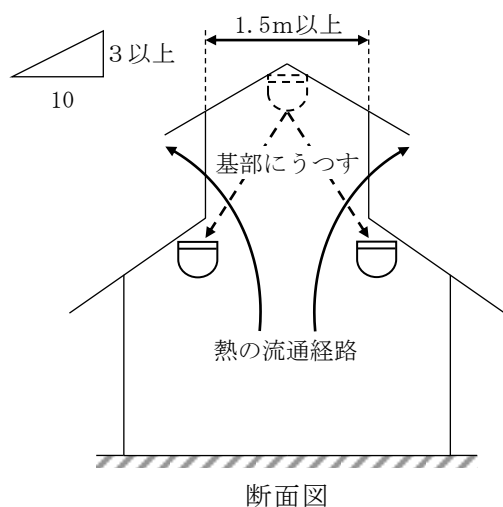
断面図 第 11-62 図
