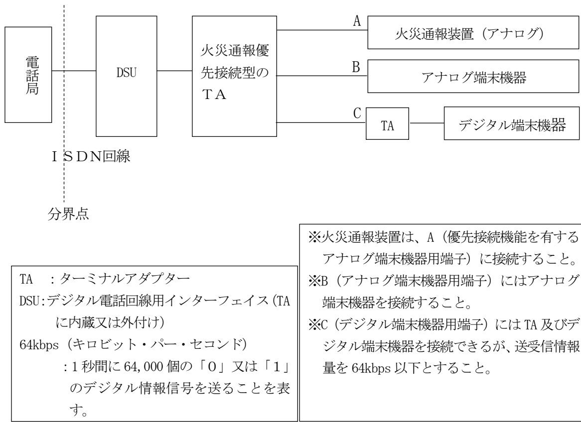
第 14-10 図 火災通報優先接続型 TA を用いた接続例
