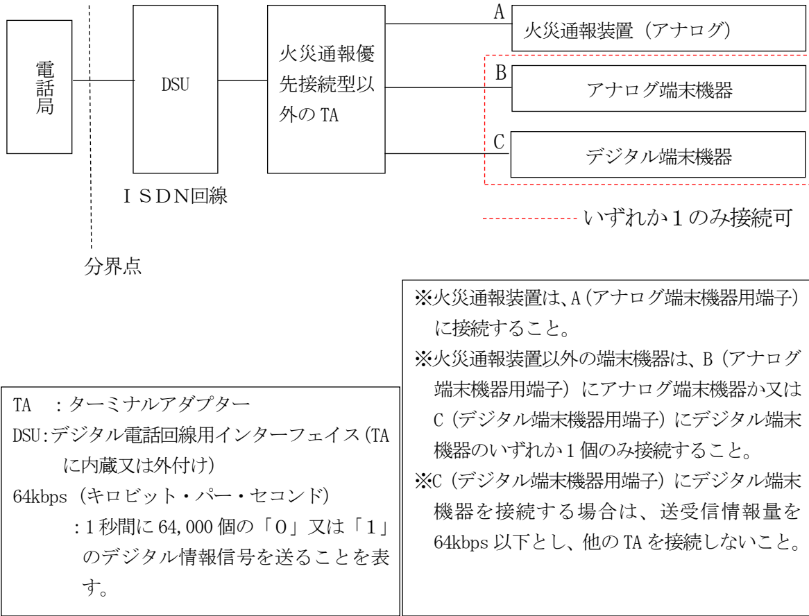
第 14-11 図 火災通報優先接続型 TA 以外の TA を用いた接続例
