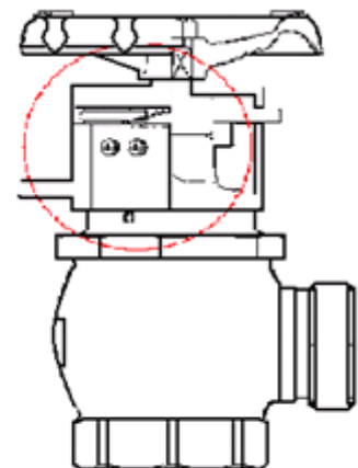
易操作性 1 号消火栓、2 号消火栓又は 広範囲型 2 号消火栓の遠隔起動部
