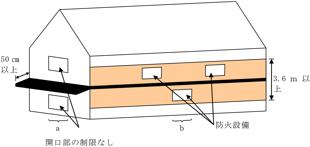
(立面図)
