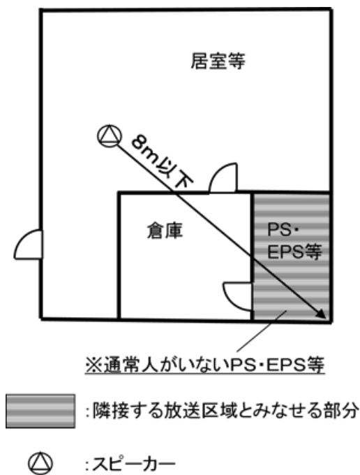
第15－7－2図（隣接していない放送区域がある場合）
